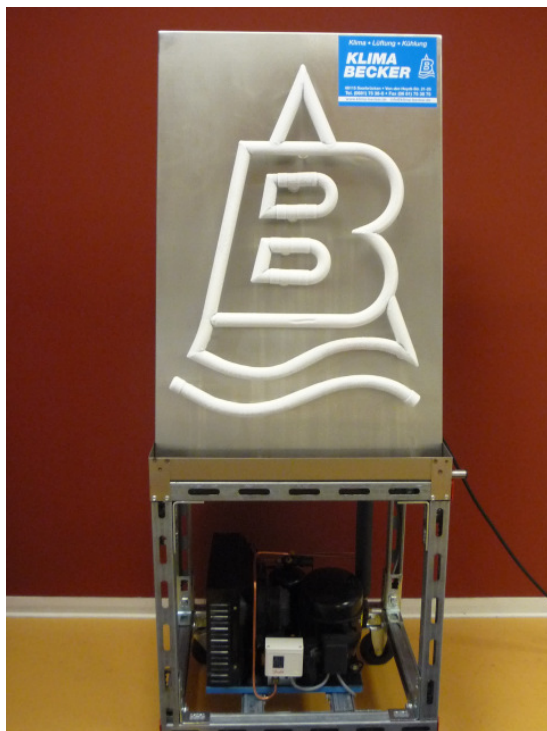
Projekt eines Auszubildenden mit besonderem Merkmal: Der Verdampfer dieser Kälteanlage hat die Form des Becker Logos, dem „Becker Eisberg“ Copyright Information: © Klima Becker
